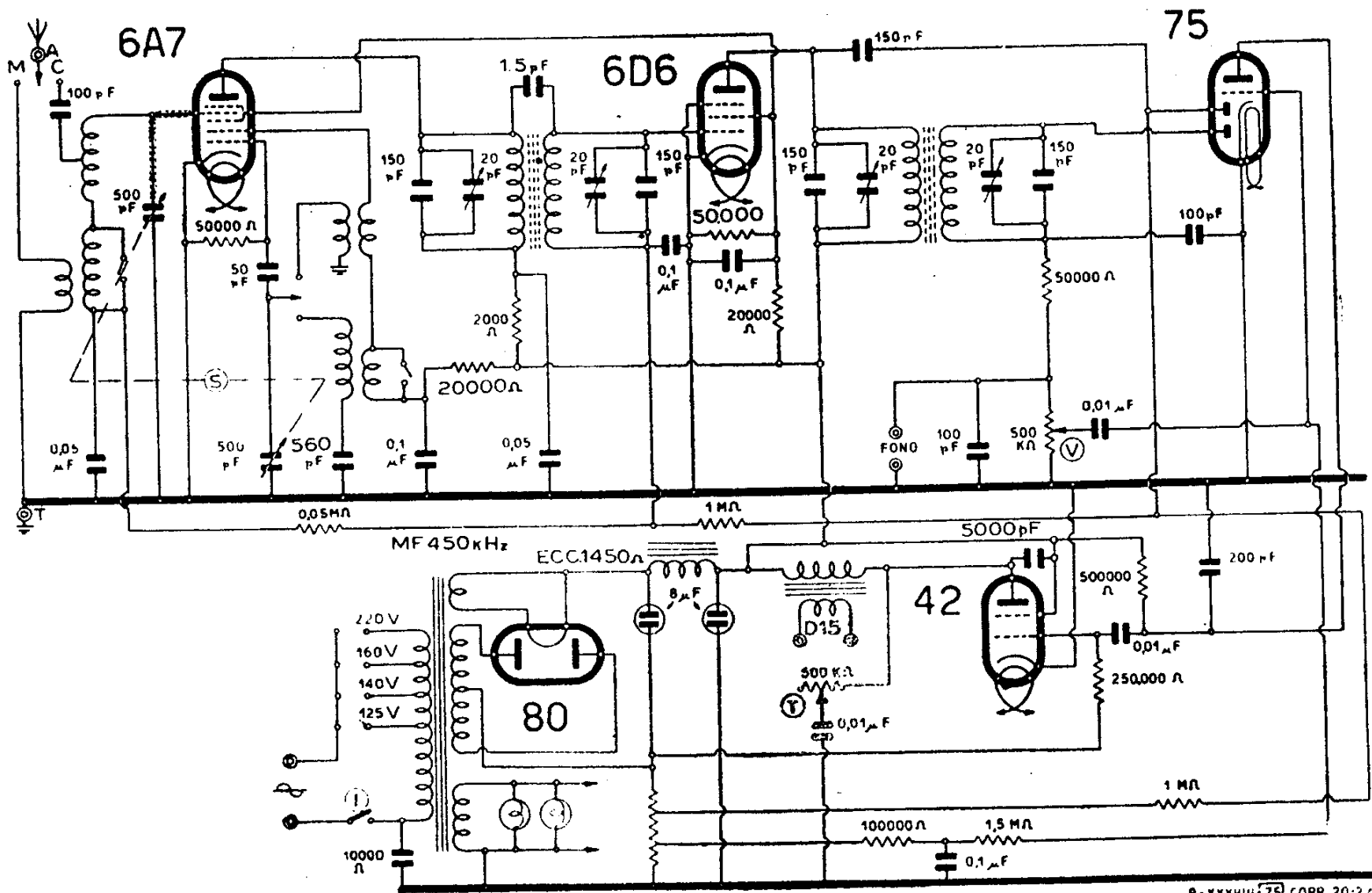
WATT RADIO - MOD. « 659 »
